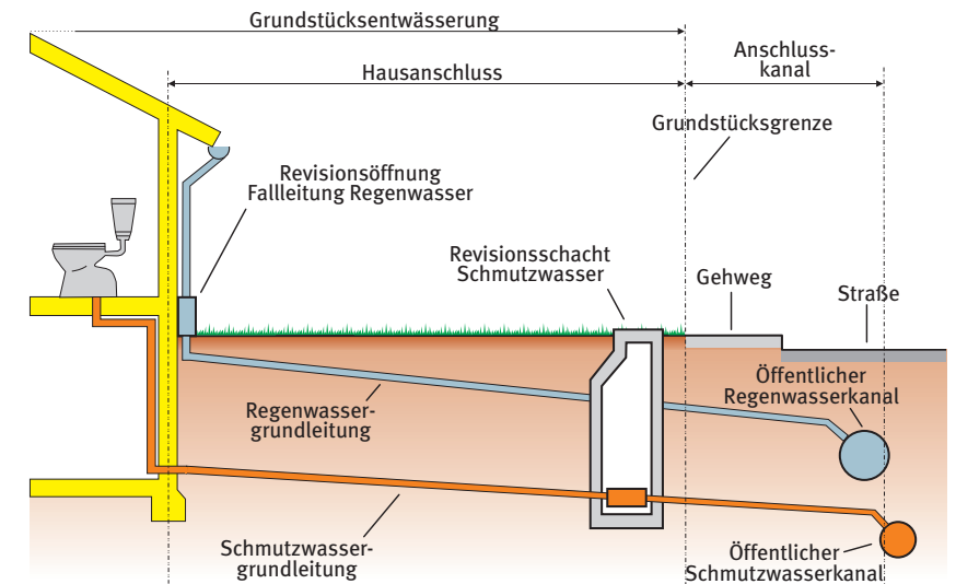
Schema einer Grundstücksentwässerung - im Trennsystem Hinweis: Anstelle der Revisionschächte sind häufig Revisionsöffnungen im Gebäude vorhanden.
